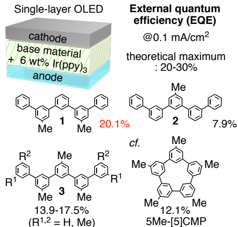
図 1: LOMP の単層 OLED 性能
