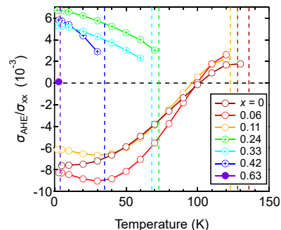
図 1 Sr 1-x Pb x RuO 3 ( 0 \leq x \leq 0.63 ) の異常ホール角の温度依存性。
