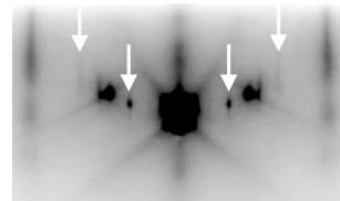
図 1, Ca インターカレートグラフェンの電子回折像。矢印はインターカレートによる周期構造由来の回折スポット。
