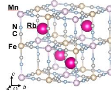
図1:室温下の \text{Rb}_{0.97}\text{MnFe} の結晶構造
