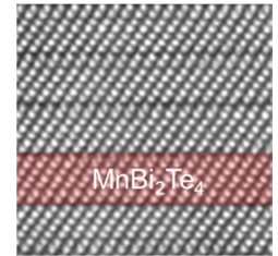
図 1: \text{MnBi}_2\text{Te}_4 薄膜
