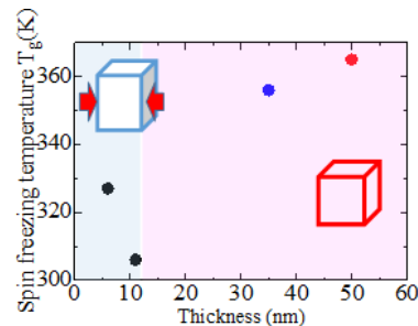
図 1. LFCG 薄膜におけるスピン凍結温度の膜厚依存性
