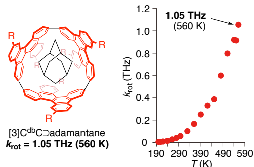
図 1: テラヘルツ回転する分子ベアリング
